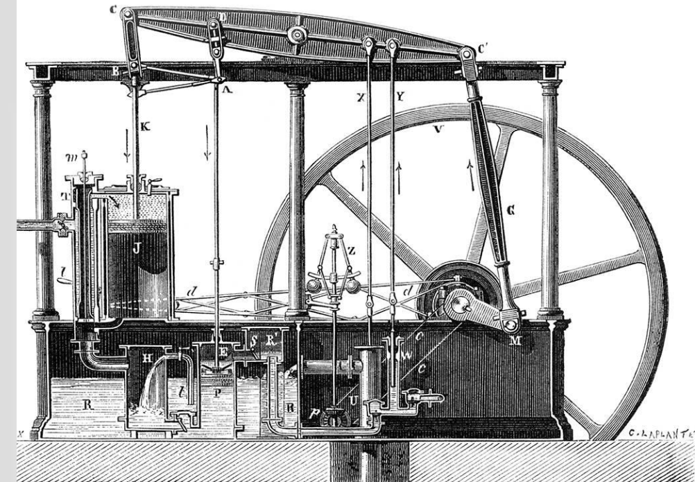
Fig. 59. — Machine à balancier de Watt.
